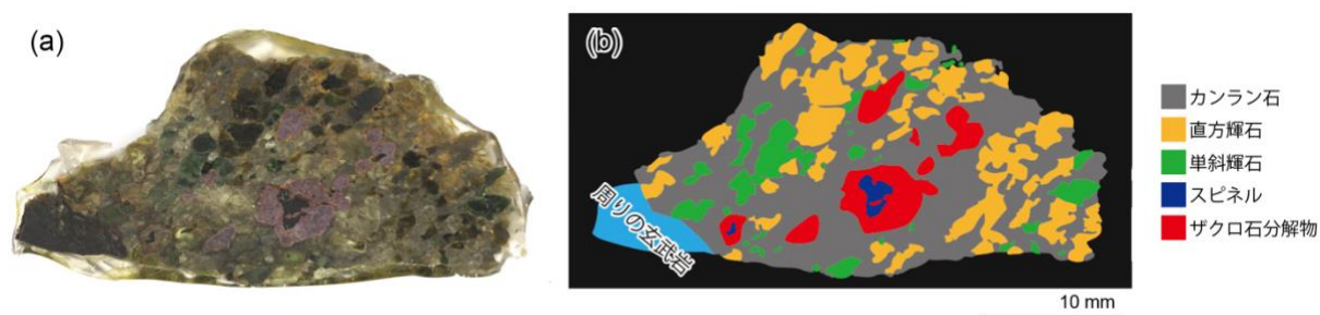
図1：アイツタキ島産のマントル捕獲岩の切断面と鉱物分布解釈図
