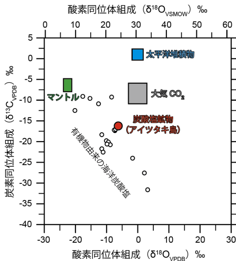
図 3：炭素・酸素同位体組成図
