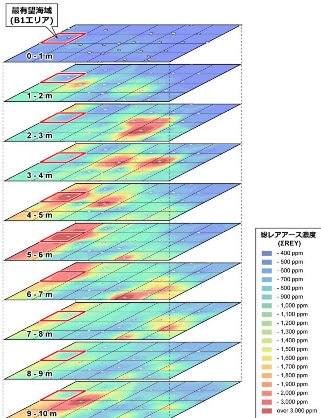
図2 有望エリアにおける海底面からの深度別レアアース濃度分布図 B1 エリア (赤枠で表示、約 105 km 2 ) が最も高い総レアアース濃度を示す。
