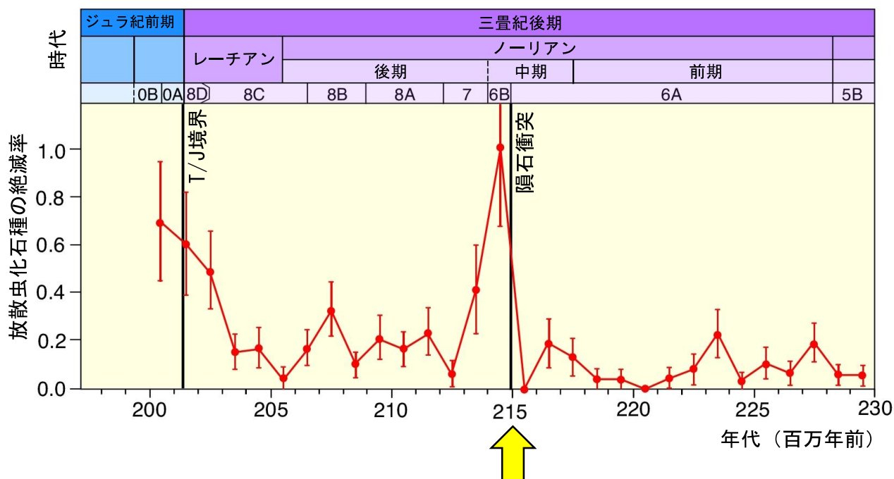
図3 三畳紀後期における放散虫の絶滅率。隕石衝突（黄色矢印）の直後に高い絶滅率を示す。ここでは、21種中18種の放散虫化石種が絶滅した。
