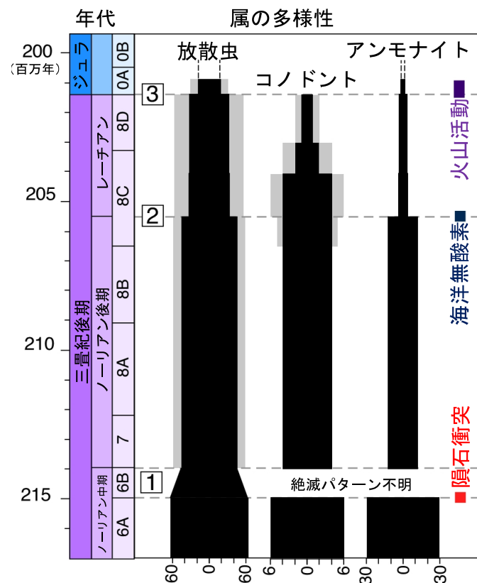
図2 三畳紀後期における放散虫、アンモナイト、コノドントの生物多様性の時代変化。三畳紀後期には大きく3回の絶滅がおこっており、このうち2億1500万年前の絶滅は、隕石衝突により引き起こされたと考えられる。
