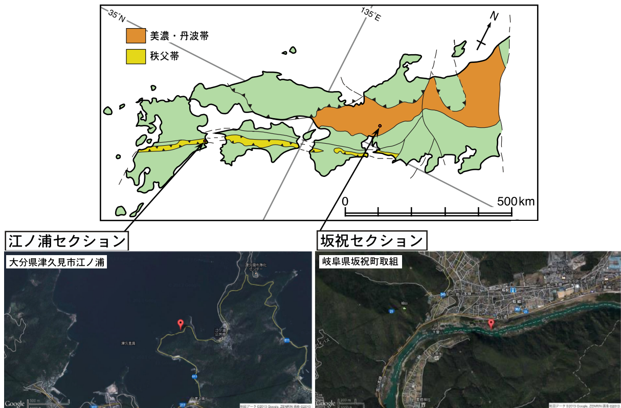
図1 これまでに2億1500万年前の巨大隕石衝突の証拠が発見された場所。研究対象は、岐阜県坂祝町の木曽川沿いに露出したチャートという岩石。
