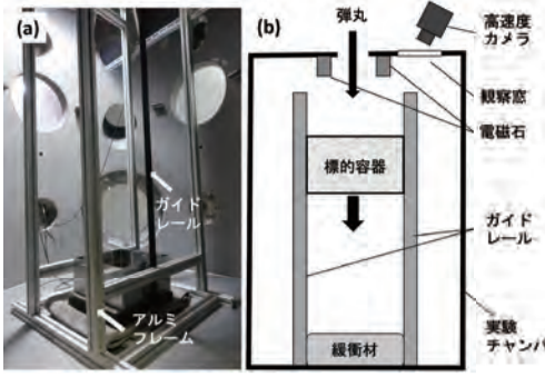
開発した低重力下での超高速衝突実験装置
